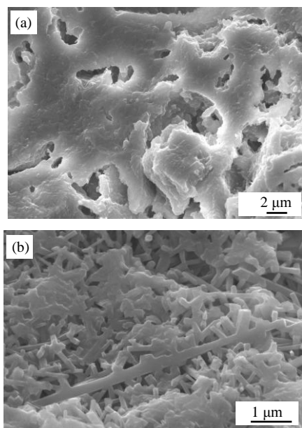
图2. 不同碳化硅/炭黑比例的35vol%料浆冷冻后坯体表面形貌
